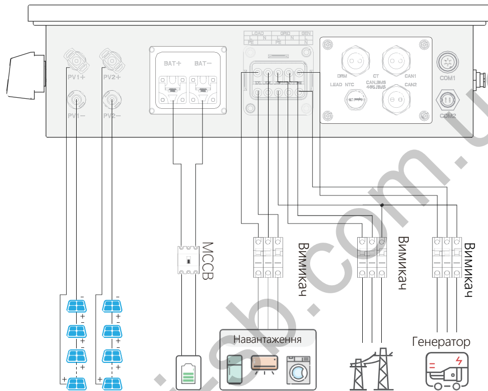
Схема електричного під'єднання для інвертора з інтерфейсом для генератора
