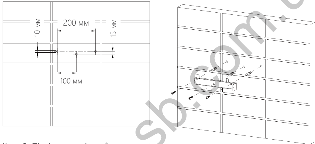
Монтаж підвісної пластини інвертора
