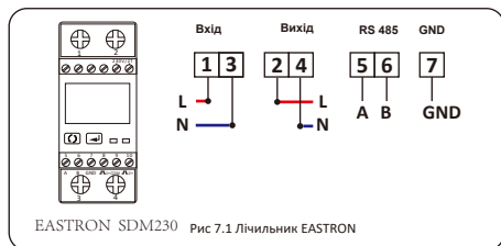
Схема підключення лічильника Easton
