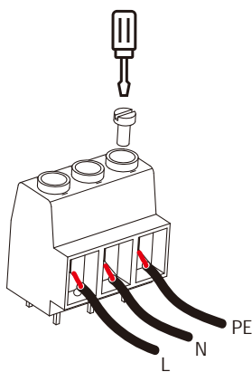
ПОРТ ГЕНЕРАТОРА
