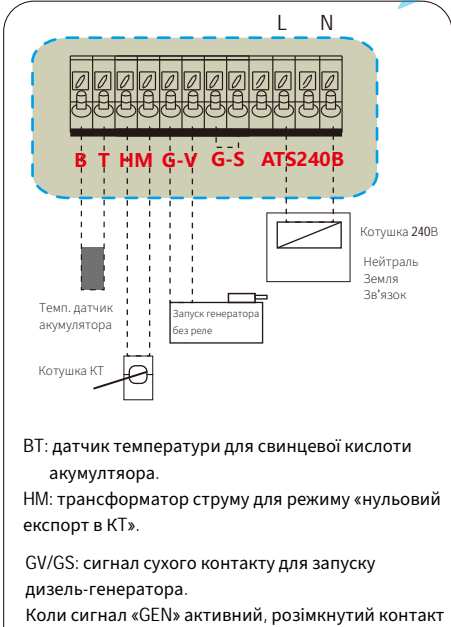
Інвертор
