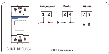
Схема підключення лічильника CHNT
