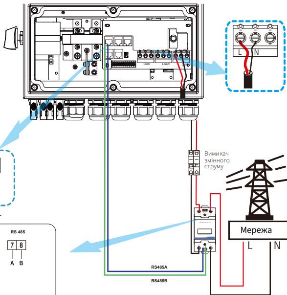
Схема підключення лічильника CHNT
