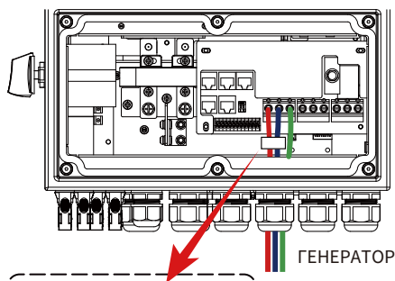
ПОРТ ГЕНЕРАТОРА
