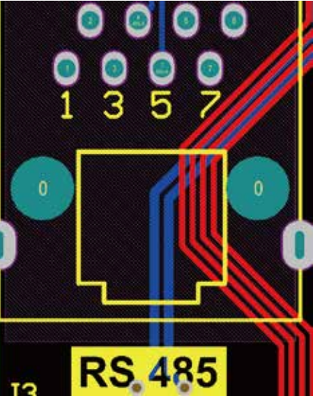
Порт RS 485
